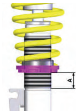
Restgewindemaß A bei Federbeinen
